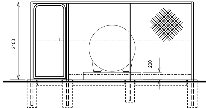
END ELEVATION
